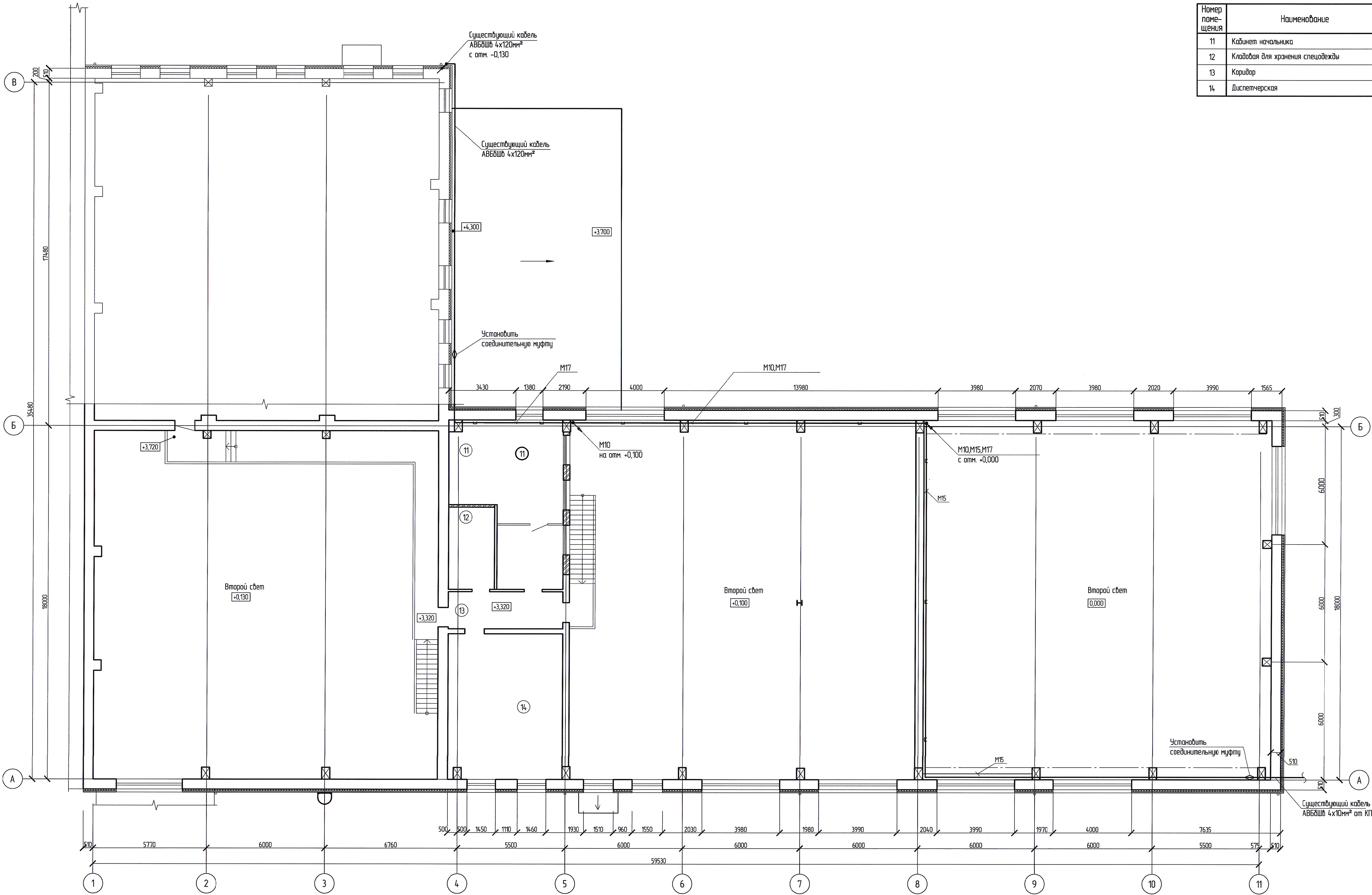
Экспликация помещений 2 этажа
