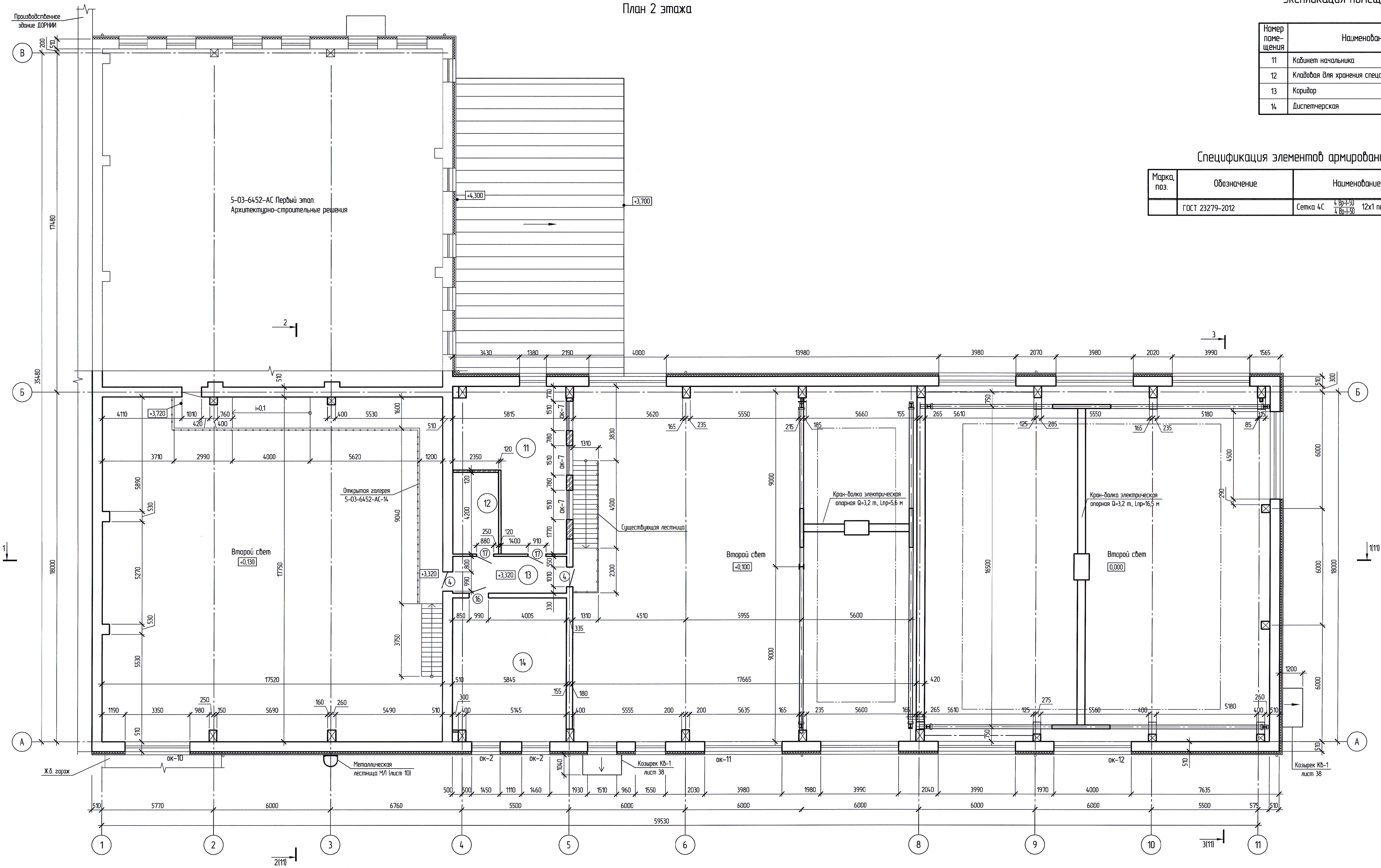
План 2 этажа
