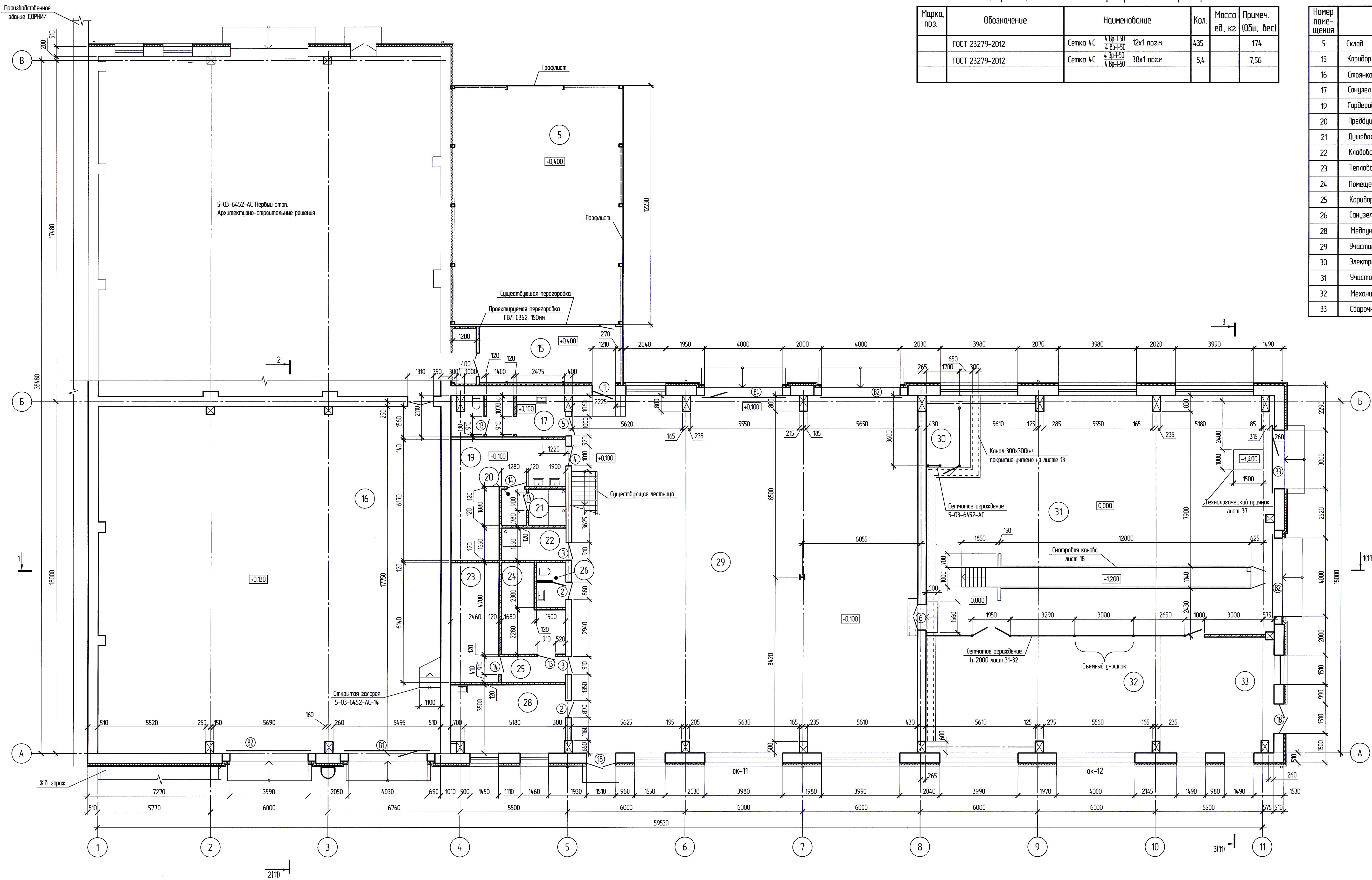
План 1 этажа
