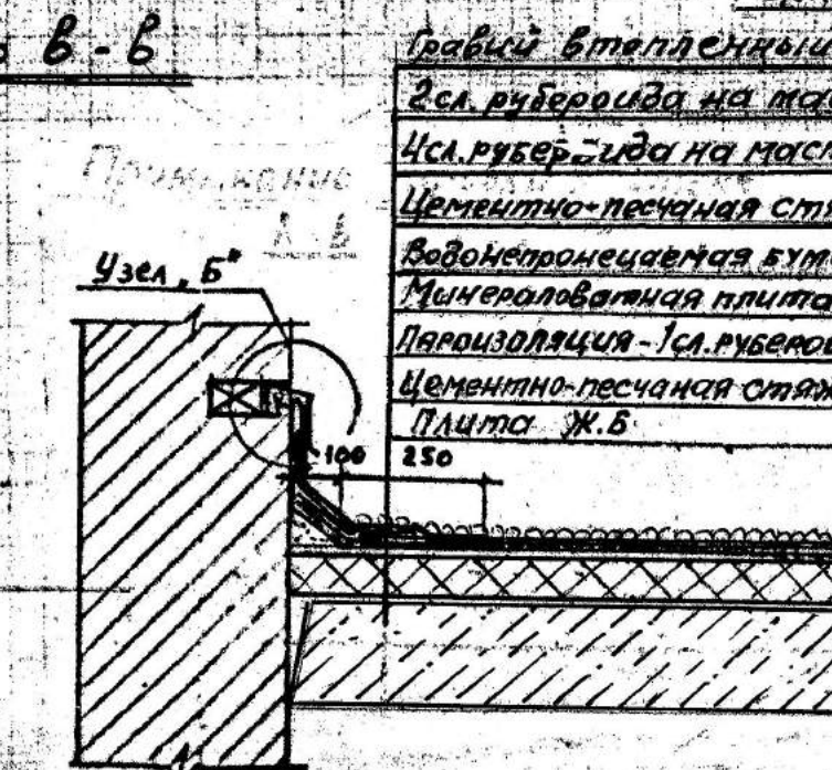
Примыкание кровли к стене
