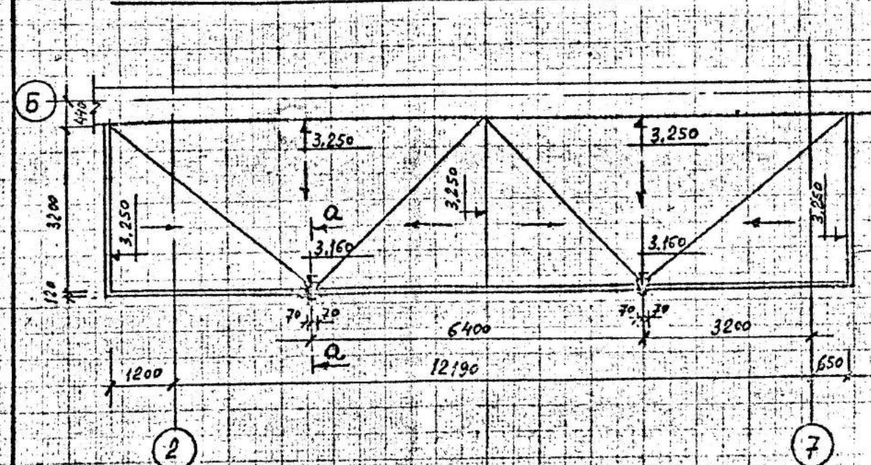
План кровли козырька главного входа.
